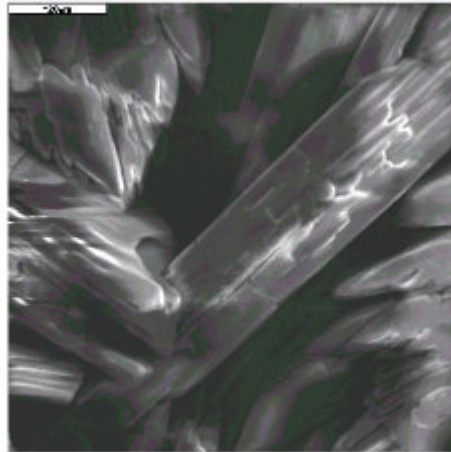
SURFACOTE 480, 1000кратное увеличение
